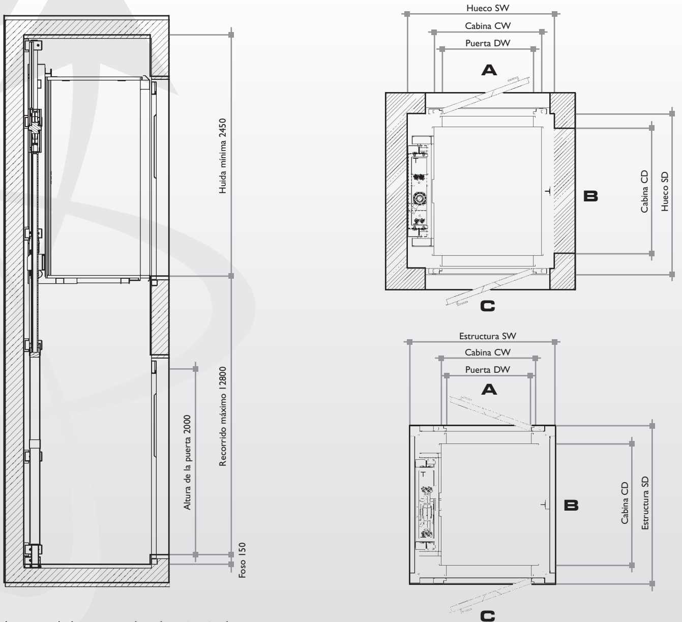
Apertura de la puerta a derecha o izquierda Dimensiones principales (en mm)
