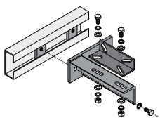
Fijaciones guías y soporte para máquinas MRL
